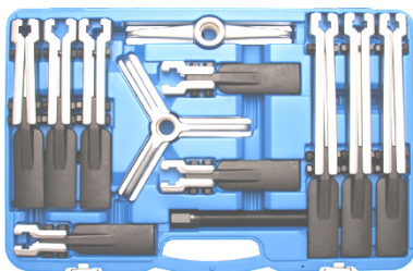
BGS7760 Trekkerset fijne bekken 2-3 armen --> Ø 135mm Jeu d'extracteurs becs fins 2-3 bras H = 105-210 & 265 mm
