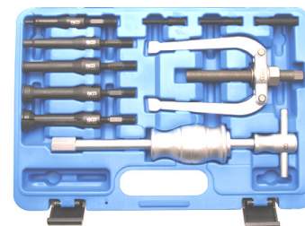
BGS7710 Trekkerset voor binnen lagere Jeu d'extracteurs de roulements intérieurs Ø 8-34mm
