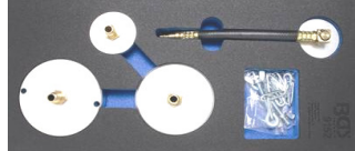
BGS9152 Adapters voor pour BGS8315 Bouchons Ø 90 Mitsubishi, Nissan, Subaru, Suzuki, Volvo S40, V40 - Ø 55 Chrysler, Ford Explorer, Hyundai, Mazda 6, Subaru - E20 Ford C-Max, Fiesta, Focus, Galaxy, S-Max 135 €
