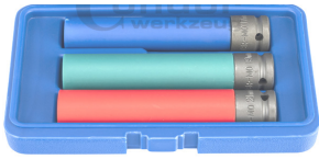
5204P XL doppen / Douilles XL 1/2 17-19-21mm voor alu velgen-jantes alu. L=150mm . Geen garantie tegen slijtage. Pas de garantie quand usées
