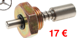
BGS8905 Blokkeerstift voor dieselpomp Calage pompe à mazout Mercedes D / TD
